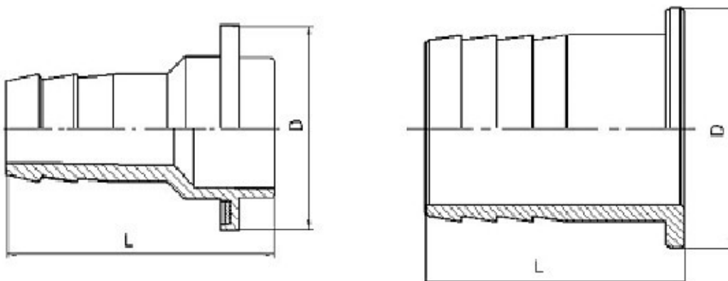
Общий вид наконечников серии НШ
