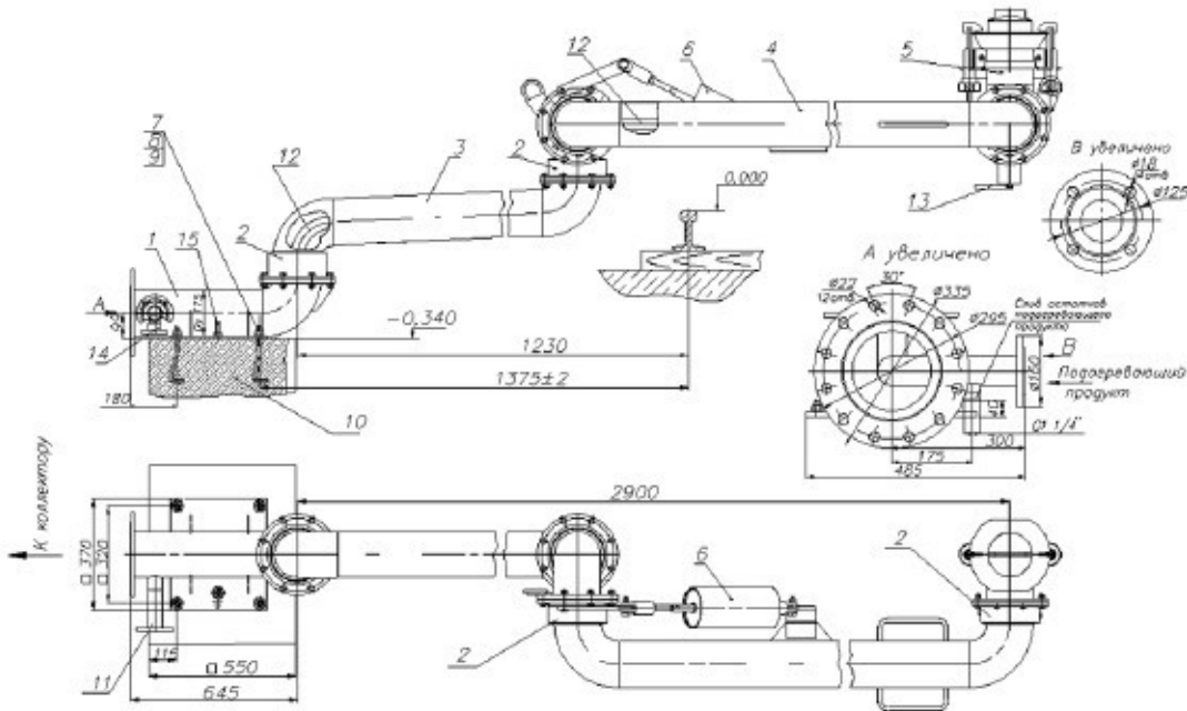
Устройство УСН-175Г
