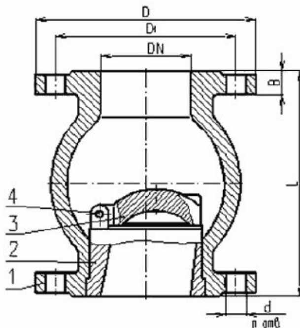
Общий вид клапана обратного ЗКО
